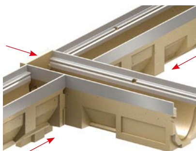
T-spoj (2 x 90°) oba žlabu napojeny do předtvarování na 0,5 m
