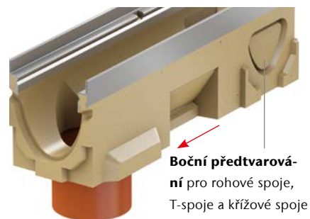
Svislý odtok pomocí otvoru ve dně s integrovaným těsněním odtoku
