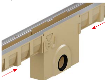
Odtok vpusť napojení linie z jedné / obou stran, vpusť obsahuje kalový koš a těsnění vodorovného odtoku
