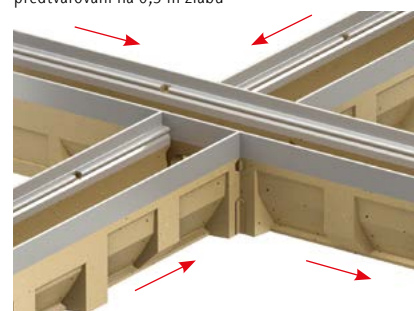
Křížový spoj (4 x 90°) žlabu napojené na průběžnou linii jsou napojeny do předtvarování na 0,5 m žlabu
